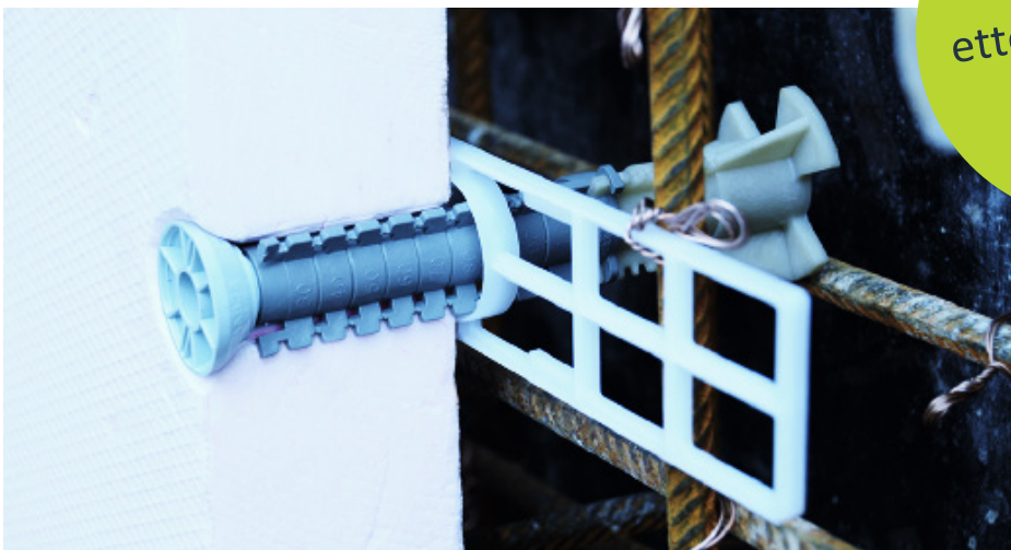
Påføring av UNI-betonghylse med beslagplate og forlengerhylse med innlagt isolasjon i forskaling.
