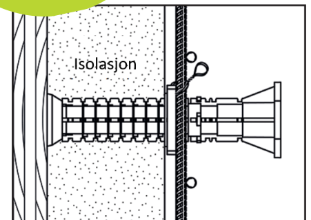
Med isolasjon i forskalingen: stikk forlengershylsen gjennom isolasjonen.
