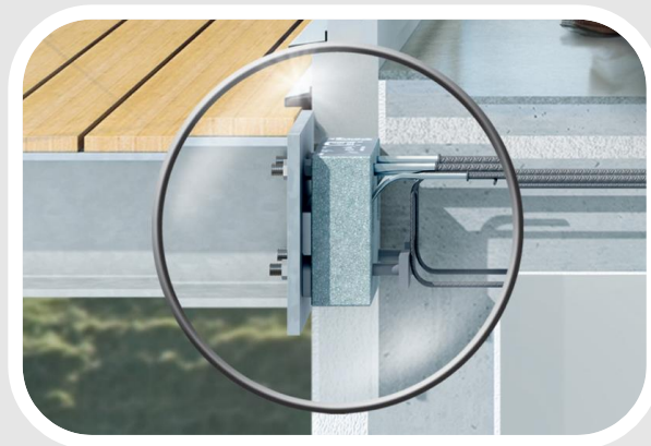
Betong til stål
